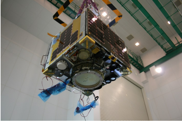
ロケット搭載前の衛星外観
