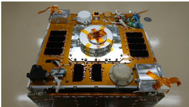
衛星トップパネル外観
