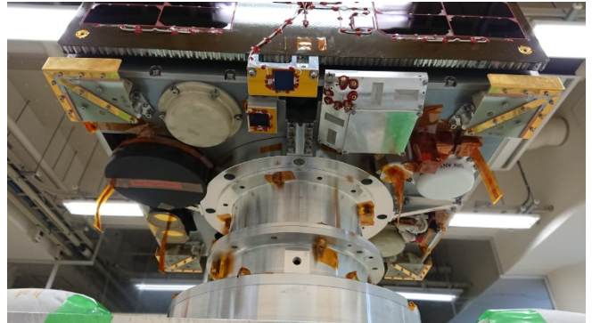
衛星ボトムパネル外観 (-X 軸)
