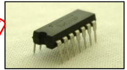
半導体LSI「74HC00」
