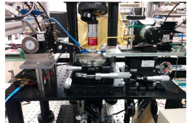
光信号→ミリ波信号 変換デバイスの測定
