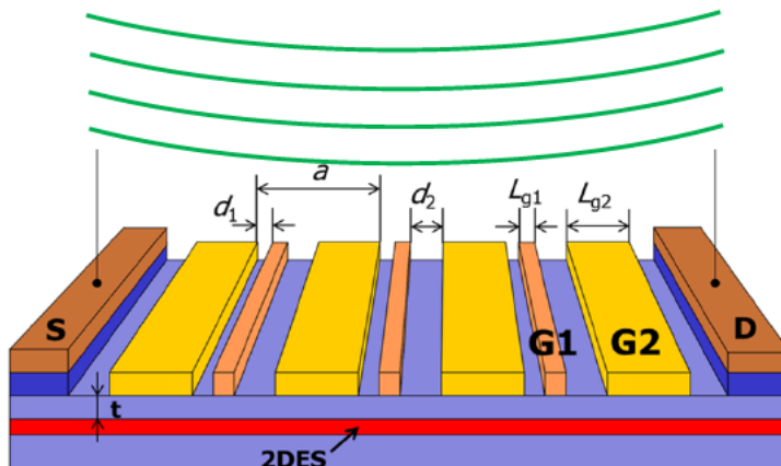
テラヘルツ波検出デバイス
