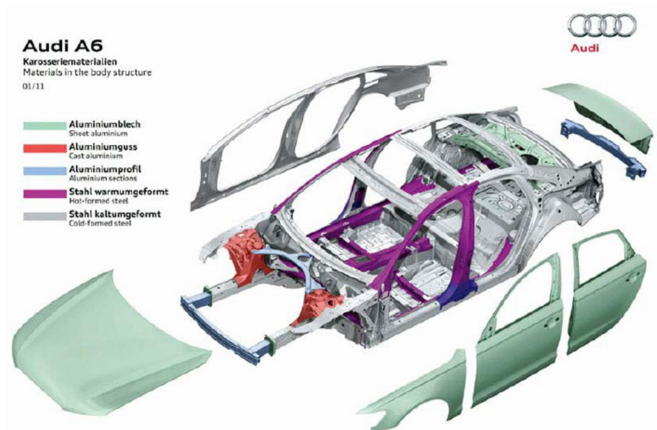
軽量化のために多用されるアルミ合金(例)
