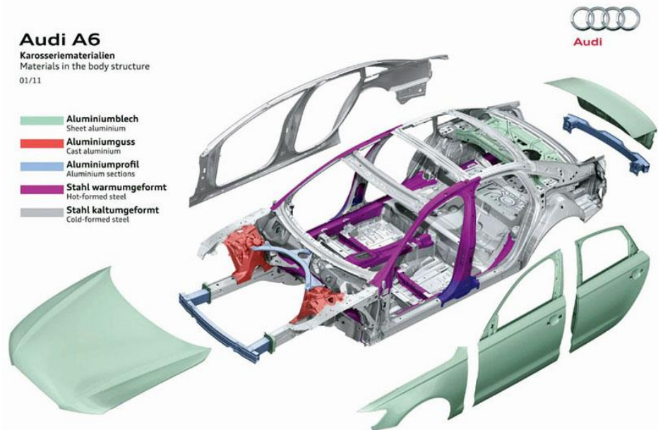
軽量化のために多用されるアルミ合金(例)
