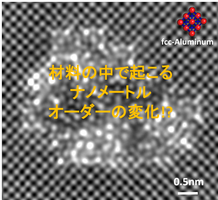
高分解能電子顕微鏡写真
