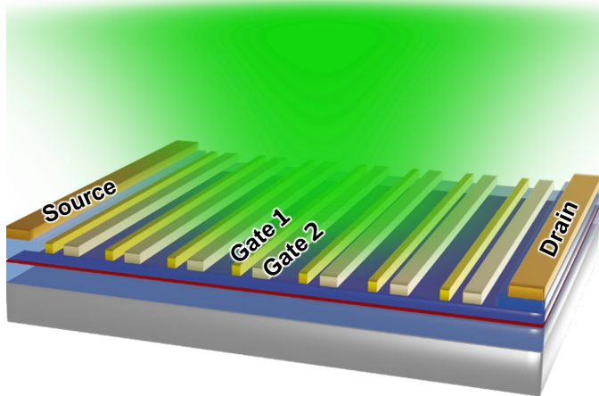
Terahertz detector
